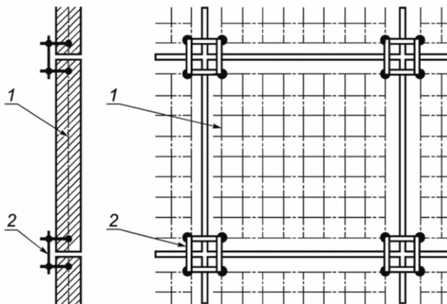
1 - сборный железобетон; 2 - проводники уравнивания потенциалов
