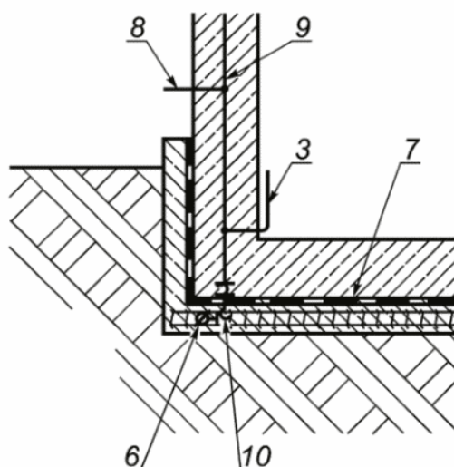
с) Соединение фундаментного заземлителя со стальной арматурой, выполненное через слой гидроизоляции
