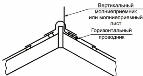
Вертикальный разрез А
