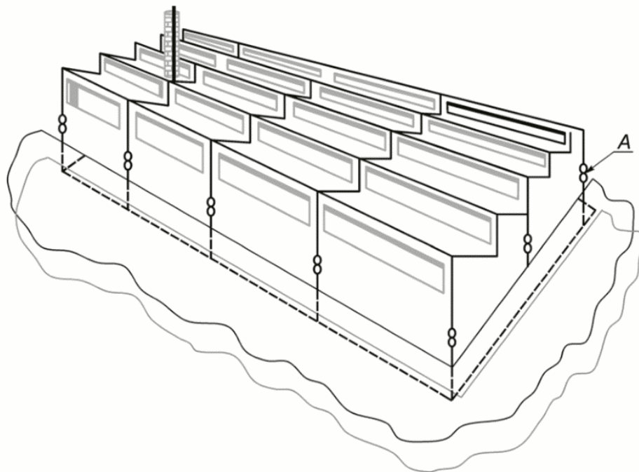
А — испытательный зажим
