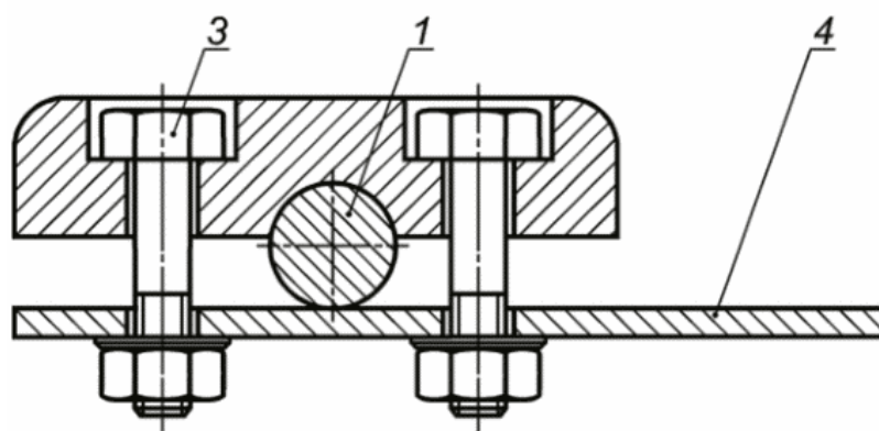
б) Проводник прямоугольного сечения с арматурным стержнем
