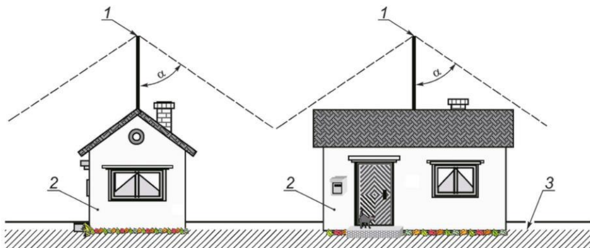
а) Пример использования одного стержневого молниеотвода
