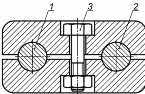
а) Круглый проводник с арматурным стержнем
