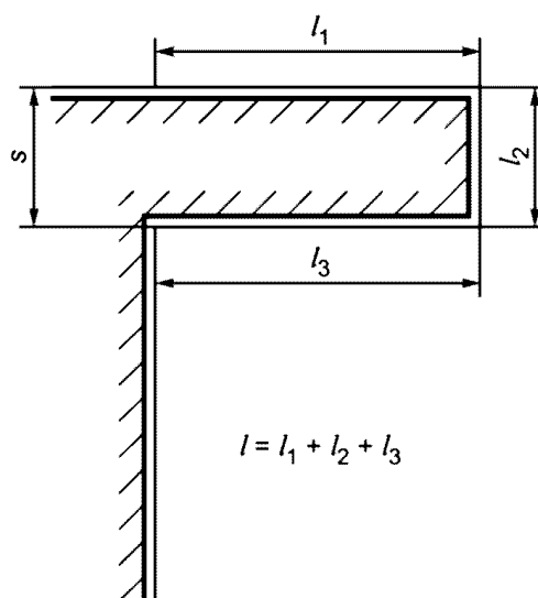
Рисунок 2 - Петля токоотвода
