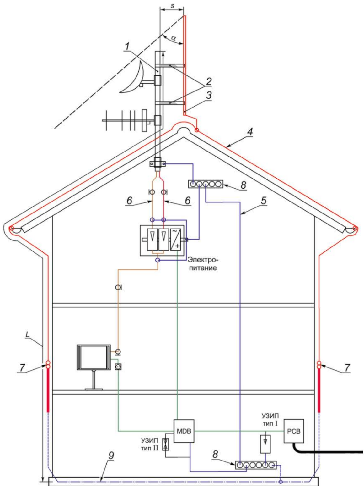
1 - металлическая опора; 2 - изолятор; 3 - стержневой молниеприемник; 4 - проводник молниеприемника; 5 - проводник уравнивания потенциалов; 6 - кабель антенны; 7 - испытательный зажим; 8 - шина уравнивания потенциалов; 9 - фундаментный заземлитель; \alpha - защитный угол; s - разделительное расстояние; l - длина для расчета разделительного расстояния; MDB - главный распределительный щит; PCB - силовая клеммная коробка
