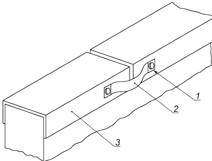
1 - соединение, устойчивое к коррозии; 2 - гибкий проводник; 3 - металлический фартук парапета
