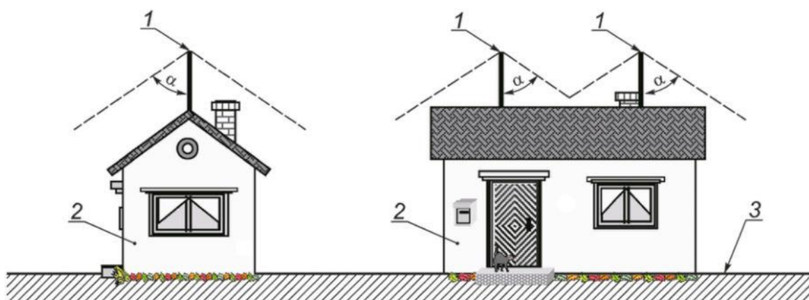
б) Пример использования двух стержневых молниеотводов
