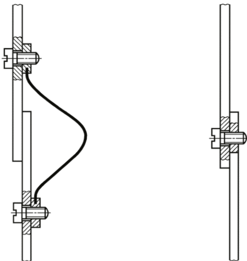
а) Перемычка гибкой металлической полосой
